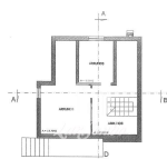
PLANTA DO SÓTÃO AL = 35,00M 2
